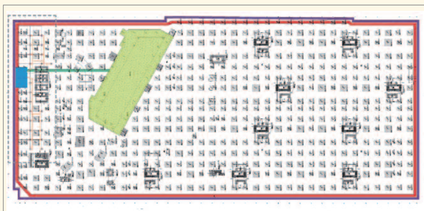
Pantallas termoactivas, en rojo, las losas termoactivas, en verde, y la sala de bombas de calor geotérmicas, azul; en los niveles subterráneos del edificio.
